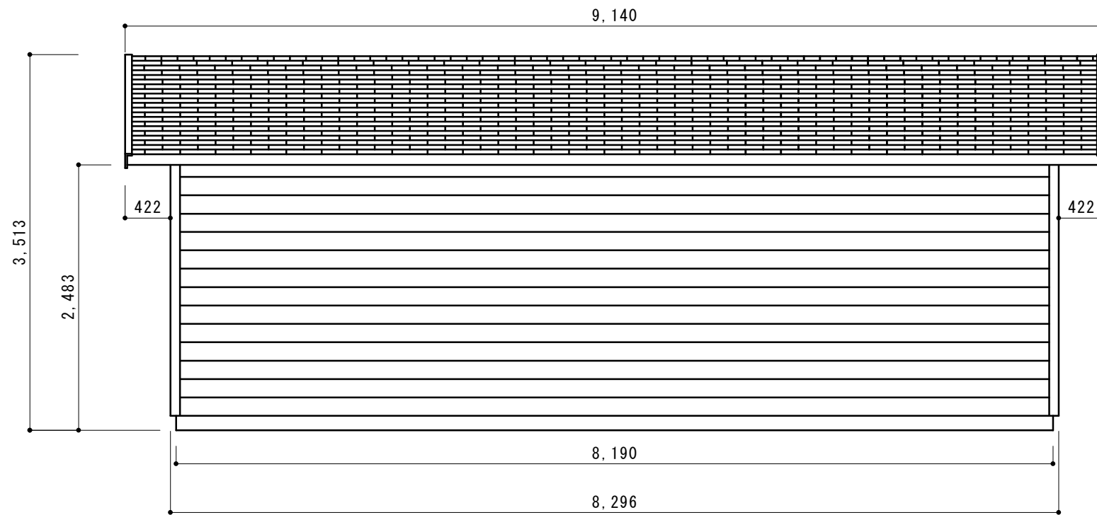
側面図
